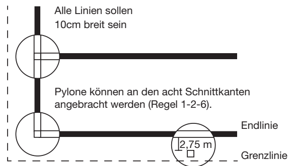
Detailausschnitt der Endzonen
